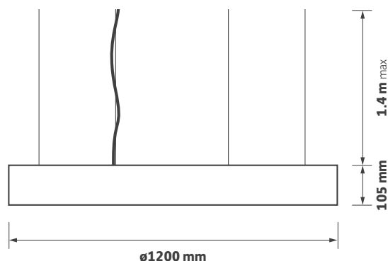
ø1200 mm
