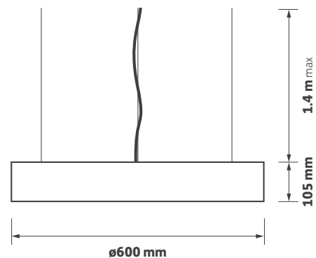
ø600 mm
